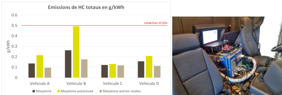
Fig. 1 : graphique - Photo : Exemple d'instrumentation avec un équipement de mesure PEMS
